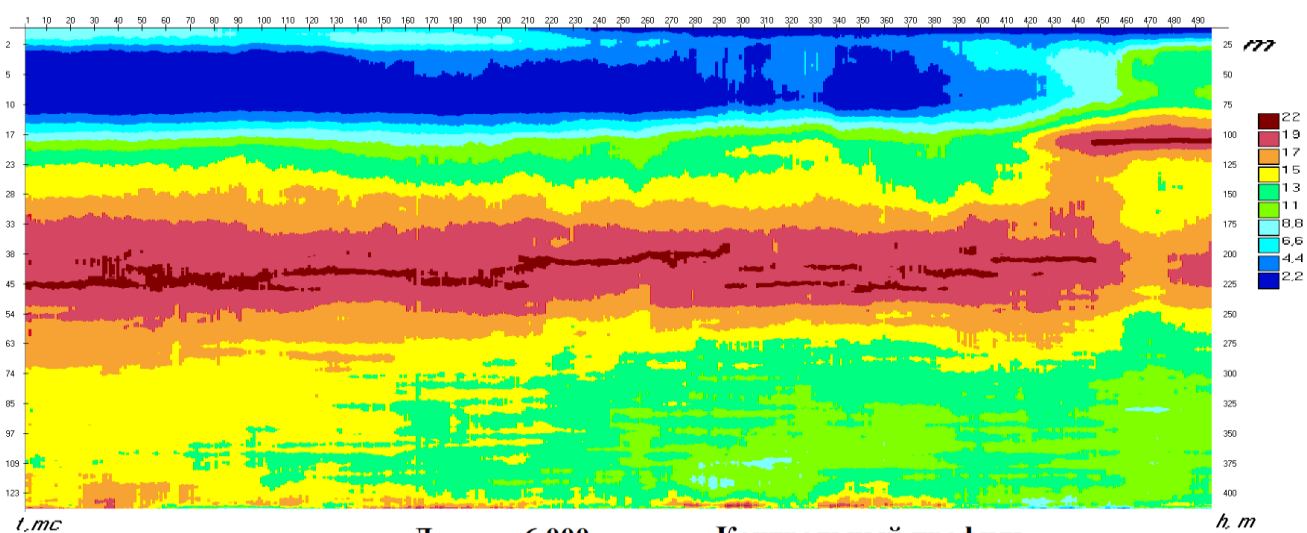
Длина - 6 000 метров. Контрольный профиль.
